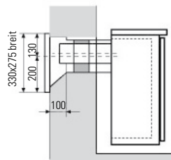
Ausführung Mauerkasten
