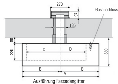
Ausführung Fassadengitter
