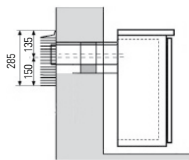
Ausführung Fassadengitter
