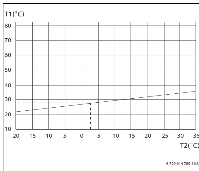
Bild 23 Fußbodenheizung
