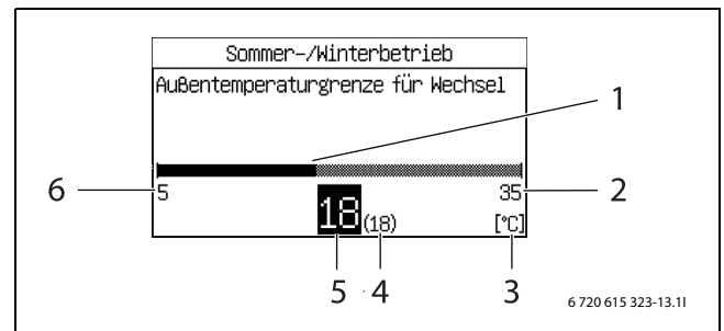
Bild 15 Hilfsinformation 2
