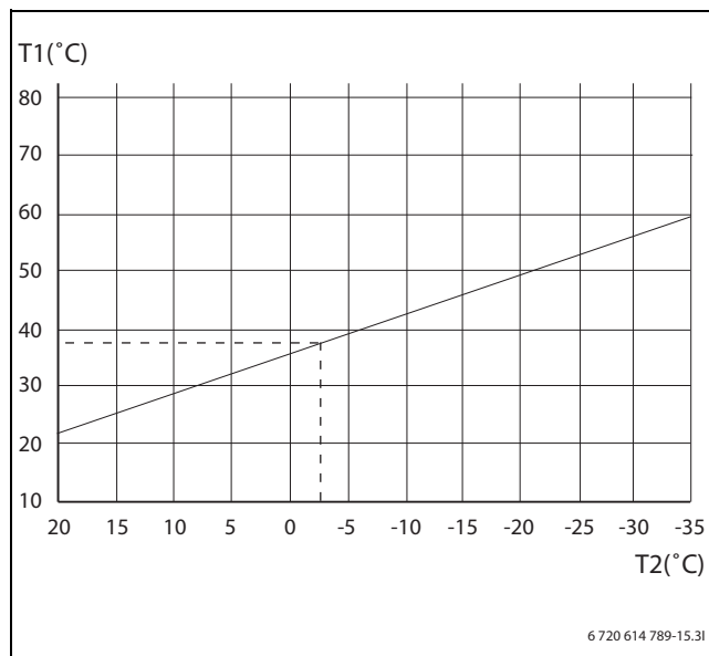
Bild 22 Heizkörper
