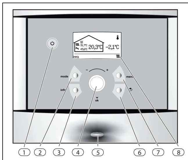
Bild 3 Bedienfeld
