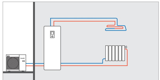
Zwei Heizkreise mit Aquarea Kombi-Hydrmodul H-Generation Ausführung „B“, ohne Pufferspeicher
