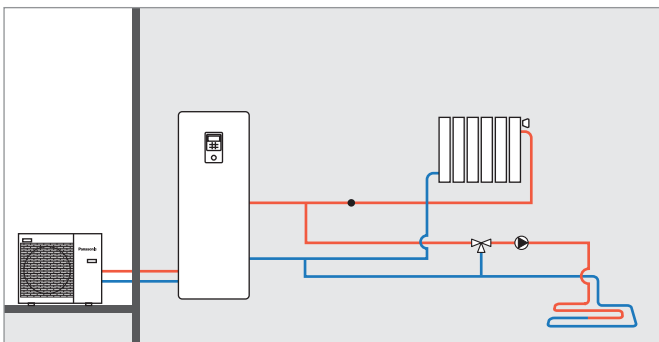
Zwei Heizkreise mit Aquarea Kombi-Hydrmodul H-Generation, ohne Pufferspeicher
