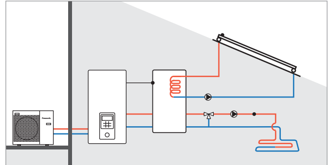
Heizungssystem mit Aquarea Splitsystem H-Generation, Pufferspeicher, Solarthermieanlage und Mischventil
