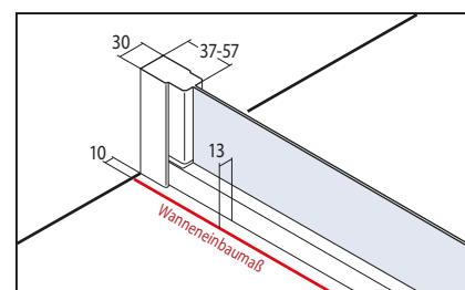
Breitenverstellung Ecke = Wanneneinbaumaß - 10
