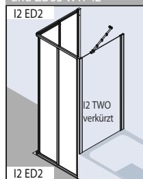
U-Kabine: I2 ED2 und I2 ED2 und I2 Seitenwand und ZDSS WTF I2
