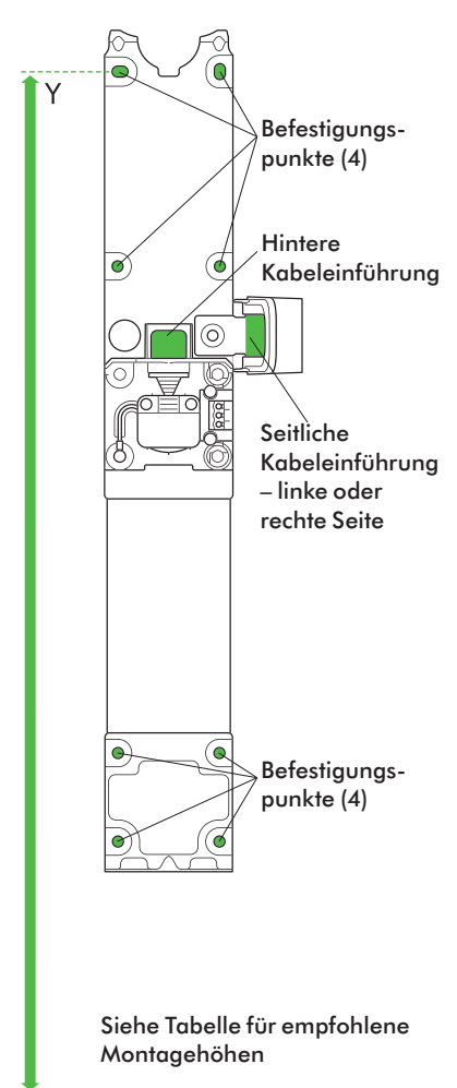
Rückplatte
