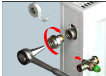
Der Anschlussnippel ist Bestandteil der RA-N Pressfit Ventile
