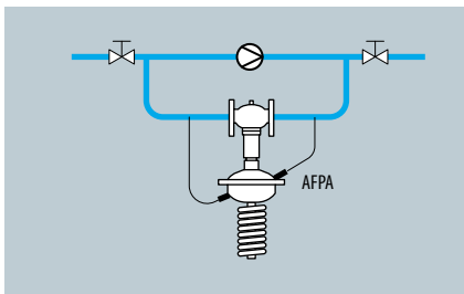
Differenzdruckregelung einer Pumpe im Bypass
