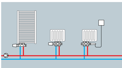
Ventileinsatz im Rücklauf
