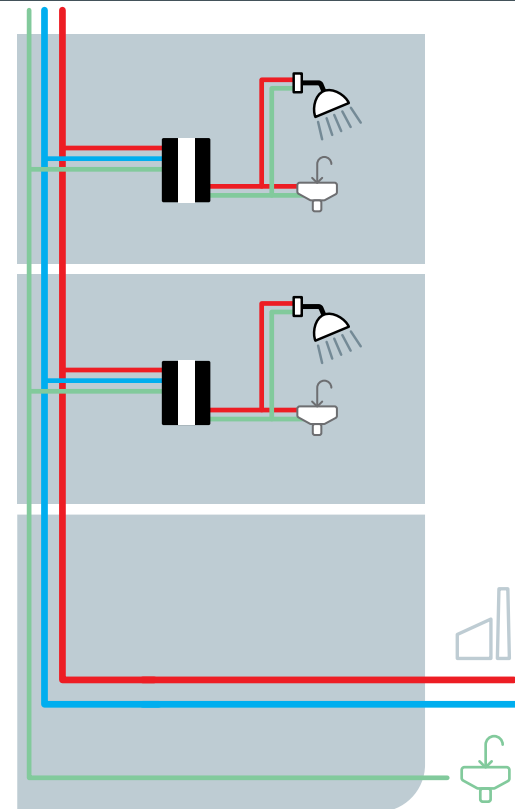
Dezentrale Trinkwassererwärmung
