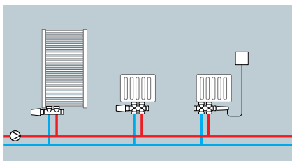
Ventileinsatz im Vorlauf
