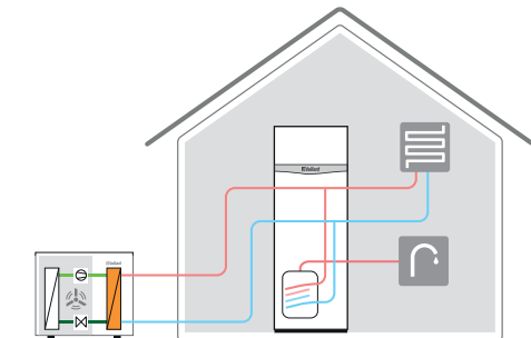
Monoblock System: alle Wärmepumpen- Komponenten in der Außeneinheit
