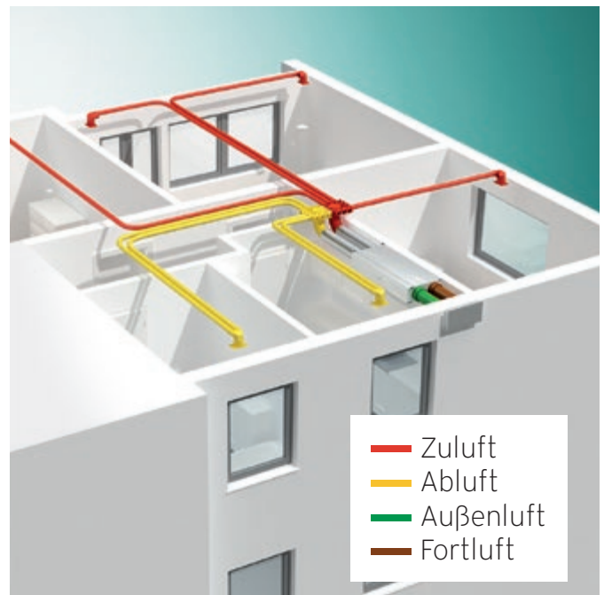
Beispielhaftes Luftkanalsystem
