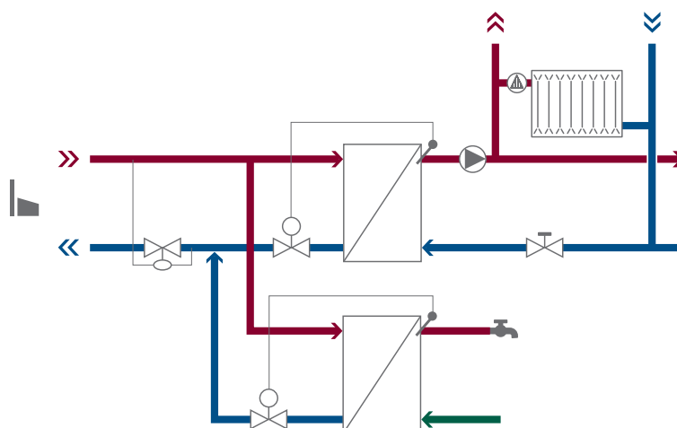
Beispiel für eine selbsttätige Regelung
