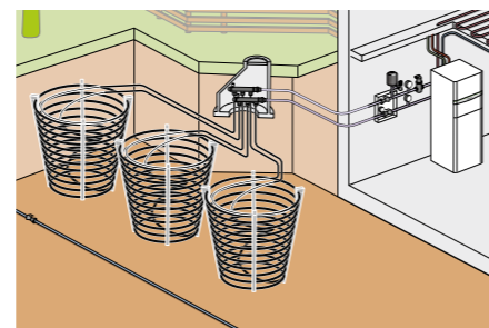
Erdwärmekörbe
