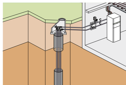
Erdsonde
