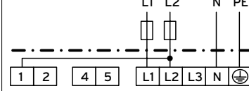
3/N/PE Einkreisumstellung - 5 7,5 kW
