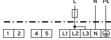
2/N/PE Boilerschaltung - 3 5,5 kW
