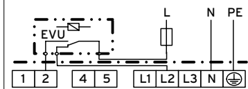
1/N/PE Zweikreisumstellung - 2* 3,5 kW / 2 kW
