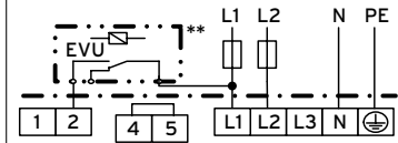
3/N/PE Zweikreisumstellung - 5 2 kW / 7,5 kW
