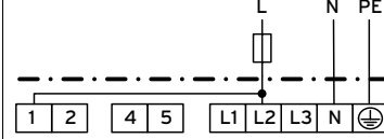
1/N/PE Einkreisumstellung - 2 4 kW
