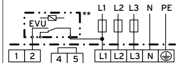
3/N/PE Zweikreisumstellung - 6 3,5 kW / 7,5 kW
