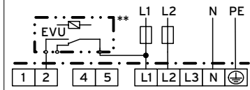
2/N/PE Zweikreisumstellung - 4 3,5 kW / 5,5 kW
