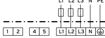
3/N/PE Boilerschaltung - 4 7,5 kW
