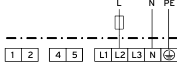
1/N/PE Boilerschaltung - 2 4 kW
