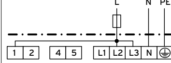
2/N/PE Einkreisumstellung - 4 5,5 kW
