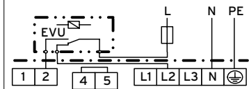
2/N/PE Zweikreisumstellung - 3 2 kW / 5,5 kW
