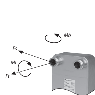
Fig. 3 Drejningsmoment / Fig. 3 Torque force / Abb. 3 Drehmoment / Fig. 3 Force de couple / Fig. 3 Esfuerzo de torsión / Fig. 3 Forza coppia / Fig. 3 Vridmoment / Fig. 3 Torsiekracht / Kuva 3 Vääntävä voima / 3 pav. Sukimo momento jėga / 3. att. Griezes momenta spēks / Joonis 3 Pöördemomendi tugevus / Obr. 3 Sila krútiaceho momentu / Slika 3 Navorna sila / SI. 3 Sila okretnog momenta / 图 3 扭力 / Фуз. 3 Въртящ момент / Slika 3 Sila obrtnog momenta / Fig. 3 Força de cuplu / 3. ábra: Azonosító címke / Obr. 3 Kroutivá sila / Rys. 3 Sila momentu obrotowego / Рис. 3 Напряжения, действующие на патрубку
