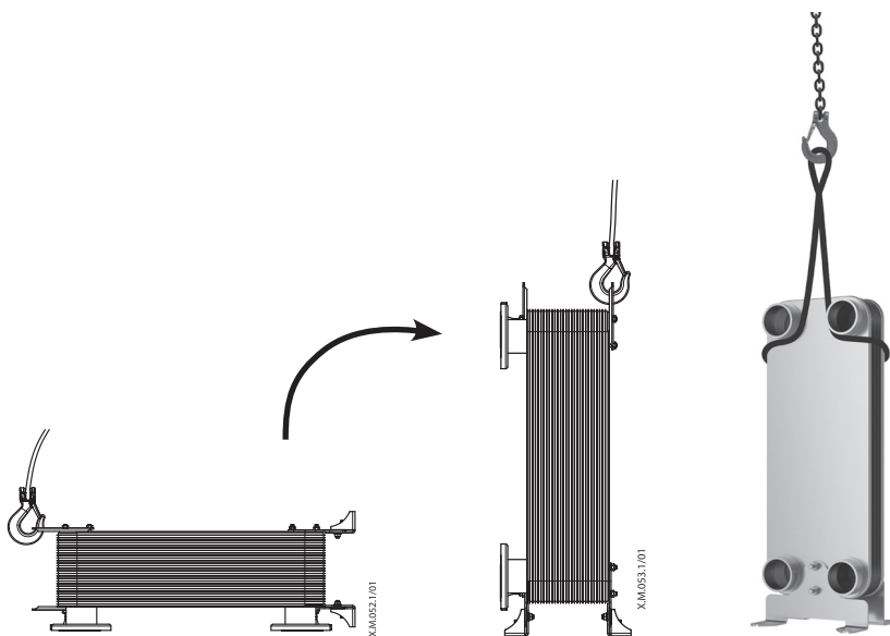
Fig. 2 Løft / Fig. 2 Lifting / Abb. 2 Heben / Fig. 2 Levage / Fig. 2 Elevación / Fig. 2 Sollevamento / Fig. 2 Lyftning / Fig. 2 Hīsen / Kuva 2 Nostaminen / 2 pav. Kėlimas / 2. att. Pacelšana / Joonis 2 Tõstmine / Obr. 2 Zdvíhanie / Slika 2 Dviganje / SI. 2 Podizanje / 图 2 起吊 / Фуз. 2 Повдигане / Slika 2 Podizanje / Fig. 2 Ridicare / 2. ábra: Emelés / Obr. 2 Zvedáni / Rys. 2 Podnoszenie / Рис. 2 Подъем
